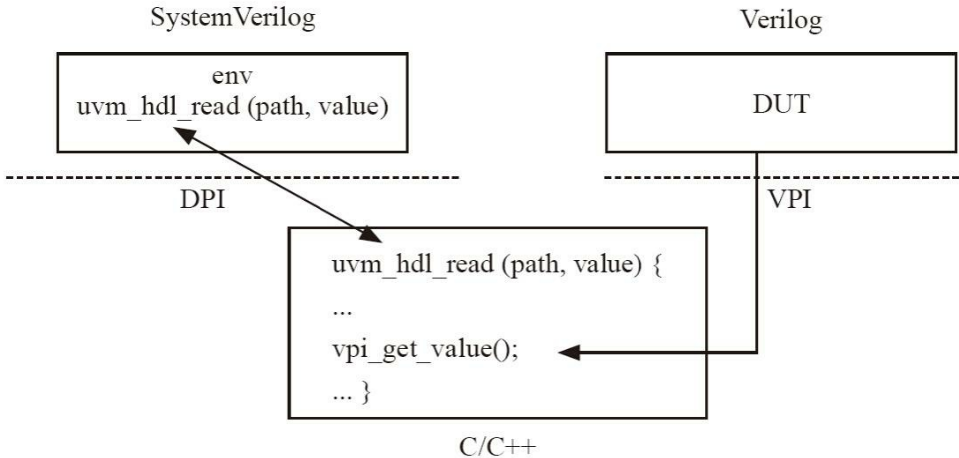
图7-6 后门访问操作原理
