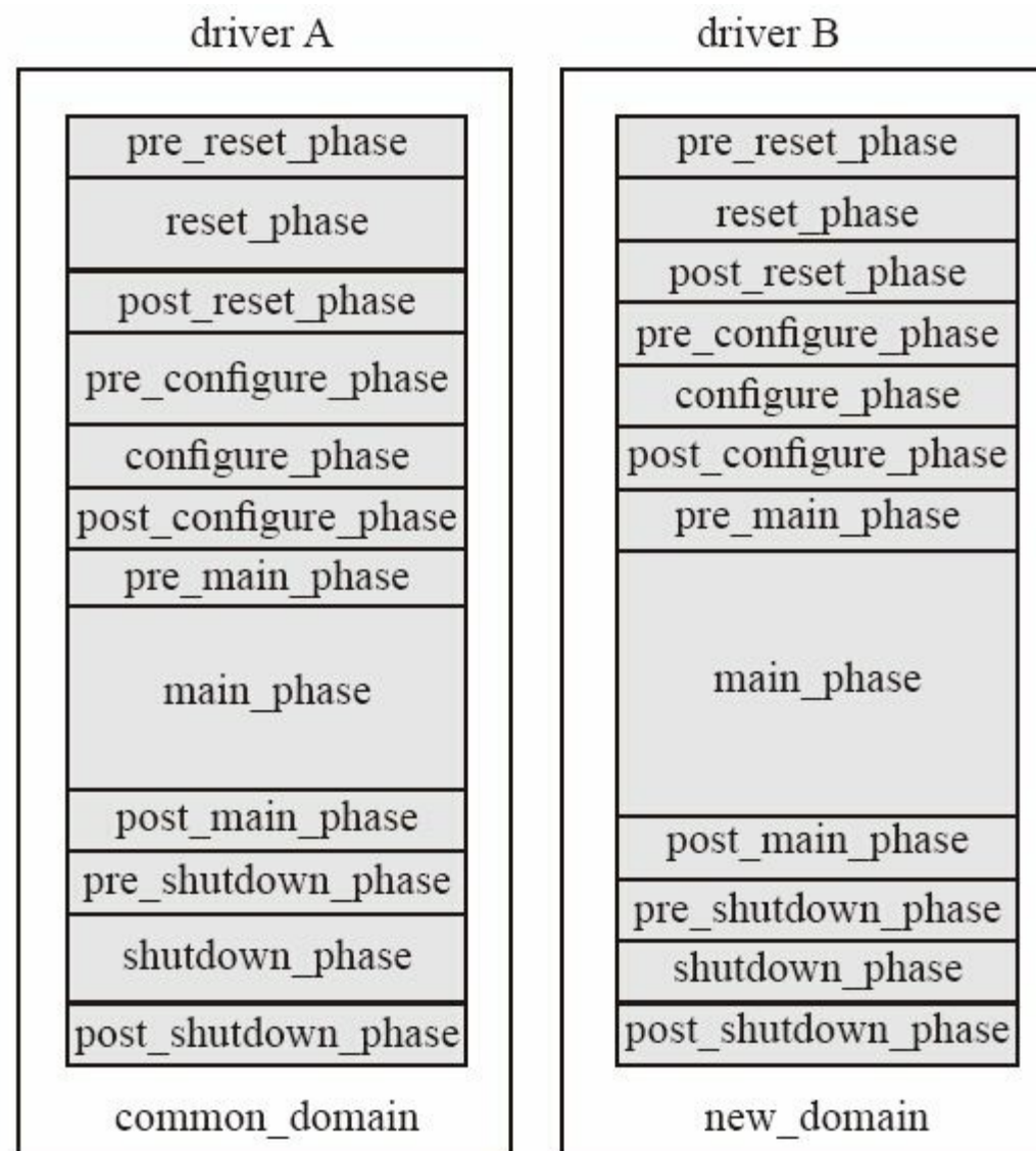
图5-7 两个driver位于不同domain
